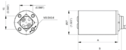
CYLINDRE EXTERNE
