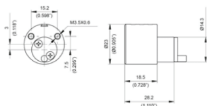
CYLINDRE INTERNE
