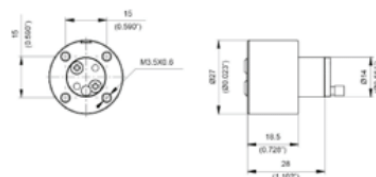
CYLINDRE INTERNE
