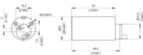
CYLINDRE EXTERNE
